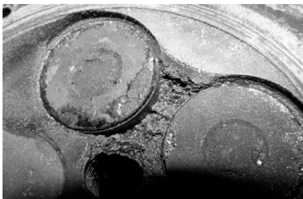
Рис.4. Камера сгорания со следами плавления стенки между седлами выпускных клапанов – номинальный режим работы ДВС (в движении).
